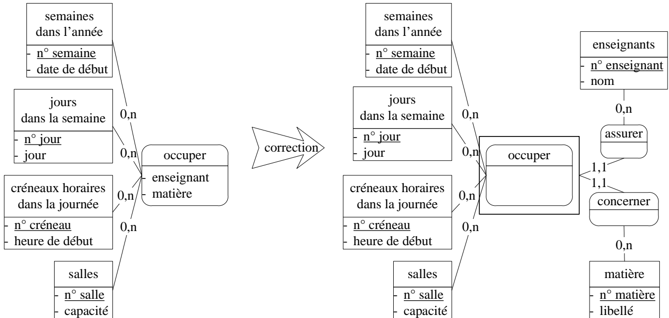
FIG. 37 – Agrégation et entités de codification
